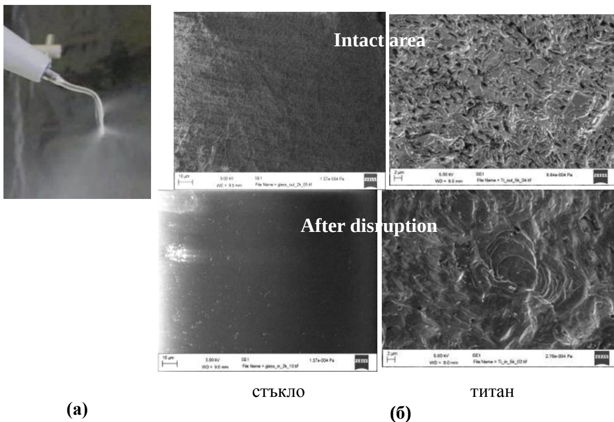
Фиг. 15 (а) Стоматологичен инструмент, използван за почистване на зъбната плака; (б) биофилми, израстнати върху стъкло (лява колона) и титан (дясна колона) и визуализирани със SEM): преди и след разрушаване посредством ефекта на кавитация (съотв. 1 и 2 ред).
